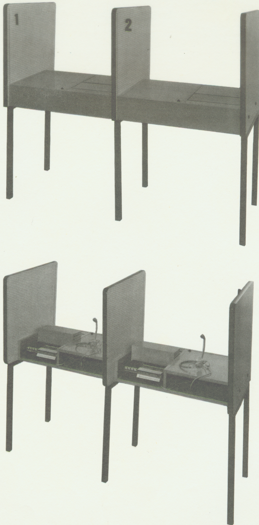
Schülertisch für Sprachlabor AAC-System mit Schülertonbandgerät EL 6940/01 und Mikrofon-Kopfhörerkombination EL 7312/11
